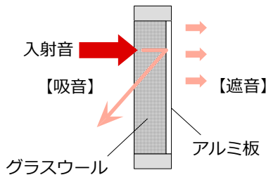
裏(遮音): アルミ複合板
